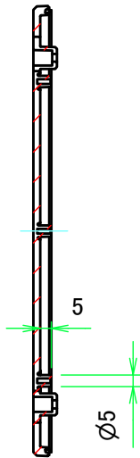
E-E ( 1 : 3 )
